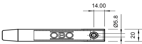
Einzelne Kabelklemme
