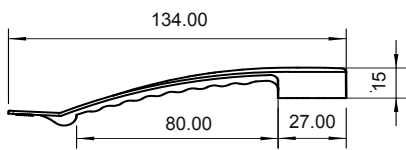
Einzelne Kabelklemme
