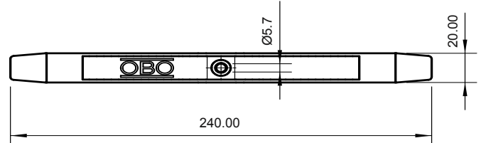
Doppelte Kabelklemme
