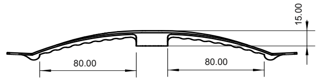
Doppelte Kabelklemme
